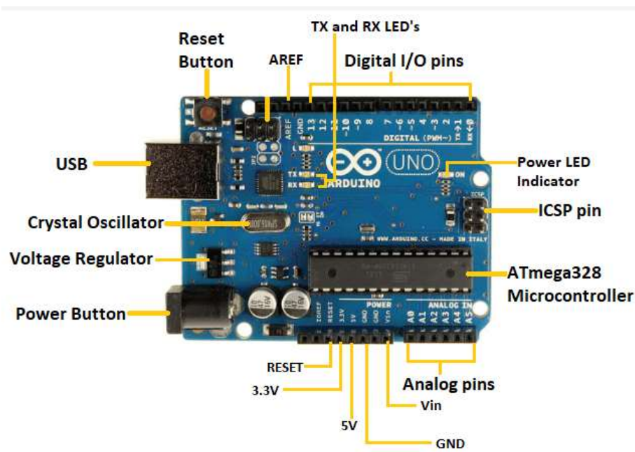
Fig: 1 Arduino board
